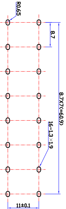
印制线路板推荐开孔尺寸
