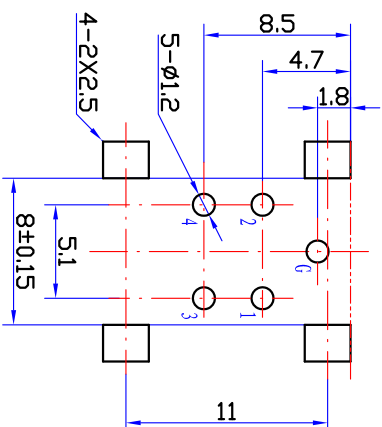
印制线路板推荐开孔尺寸
