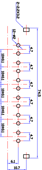
印制线路板推荐开孔尺寸
