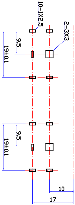
印制线路板推荐开孔尺寸
