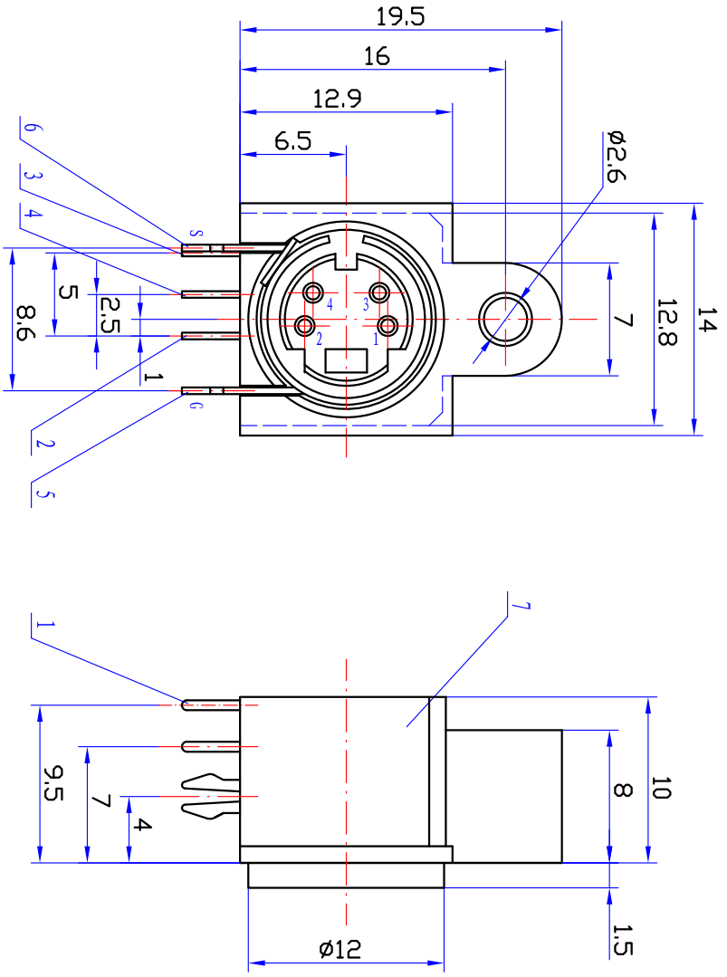
接点示意图
