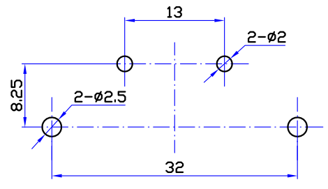
印制线路板推荐开孔尺寸
