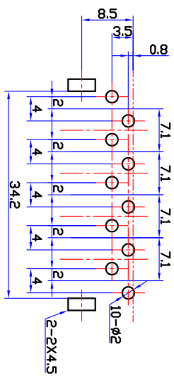
印制线路板推荐开孔尺寸
