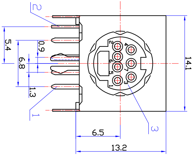
接点示意图
