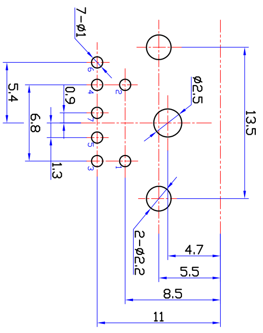
印制线路板推荐开孔尺寸 由下往上插
