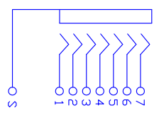
接点示意图
