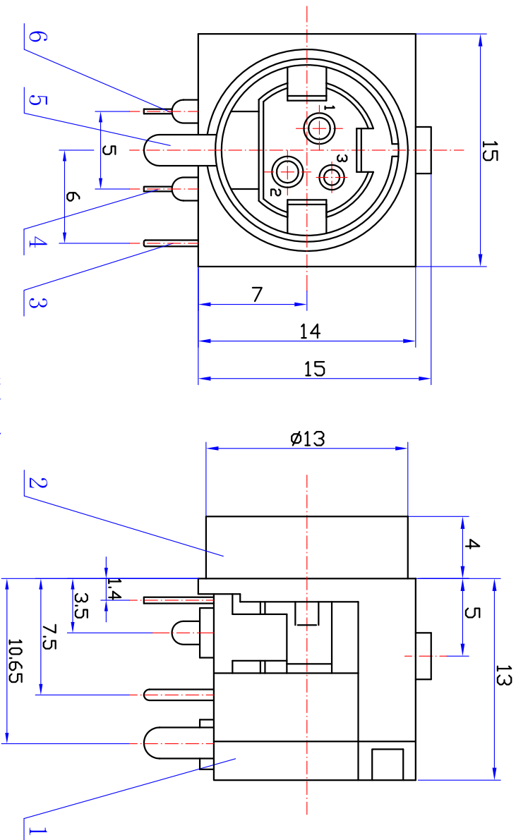
接点示意图
