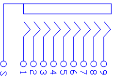
接点示意图
