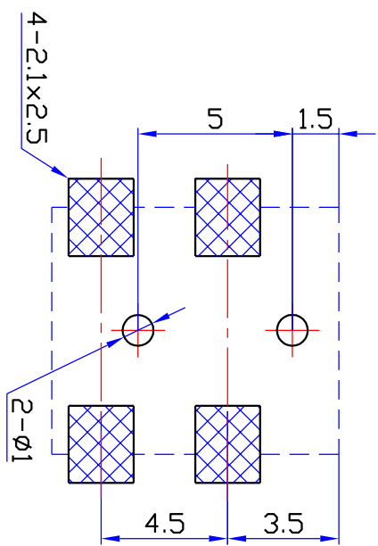
印制线路板推荐开孔尺寸
