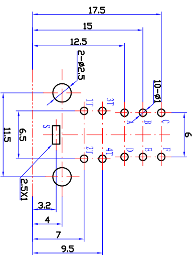
印制线路板推荐开孔尺寸
