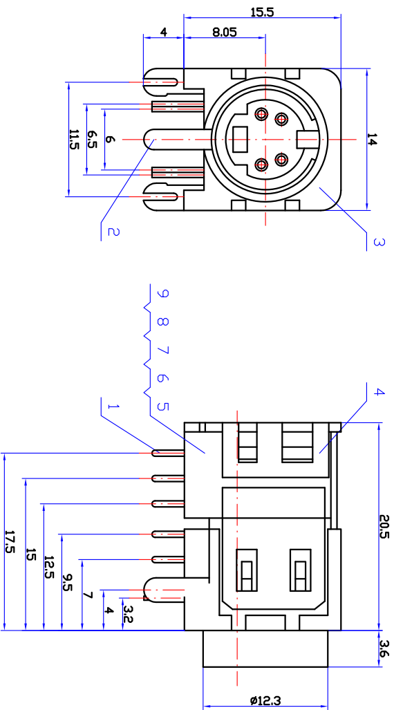
接点示意图
