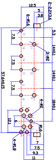
印制线路板推荐开孔尺寸 由下向上插
